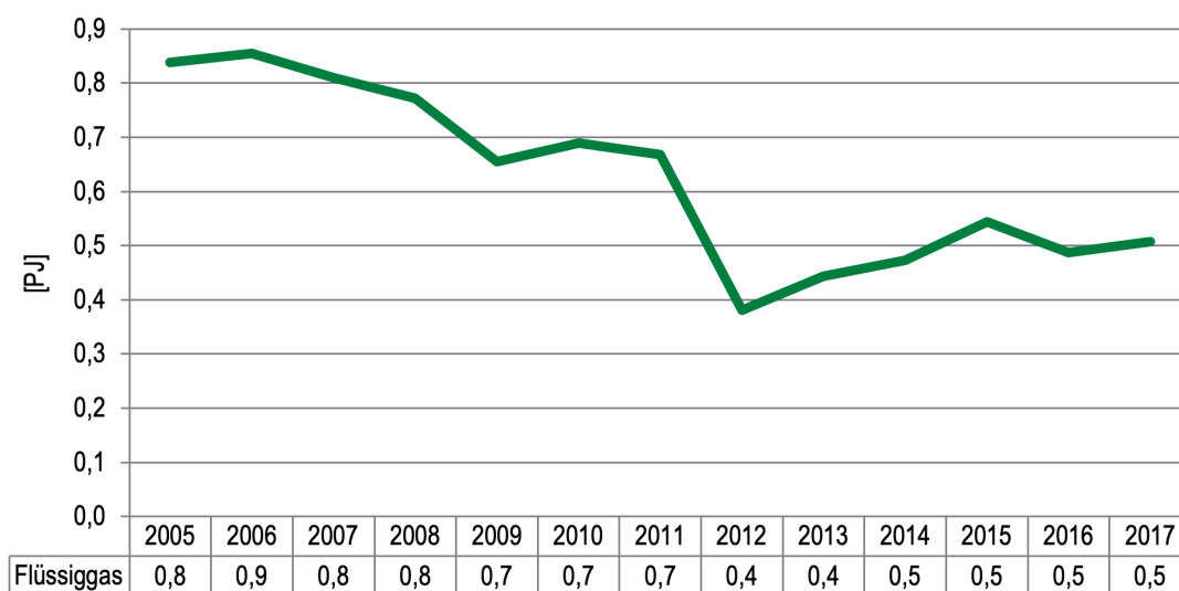
Abbildung 18: Energetischer Endverbrauch von Flüssiggas in den Jahren 2005–2017 in PJ [30]
