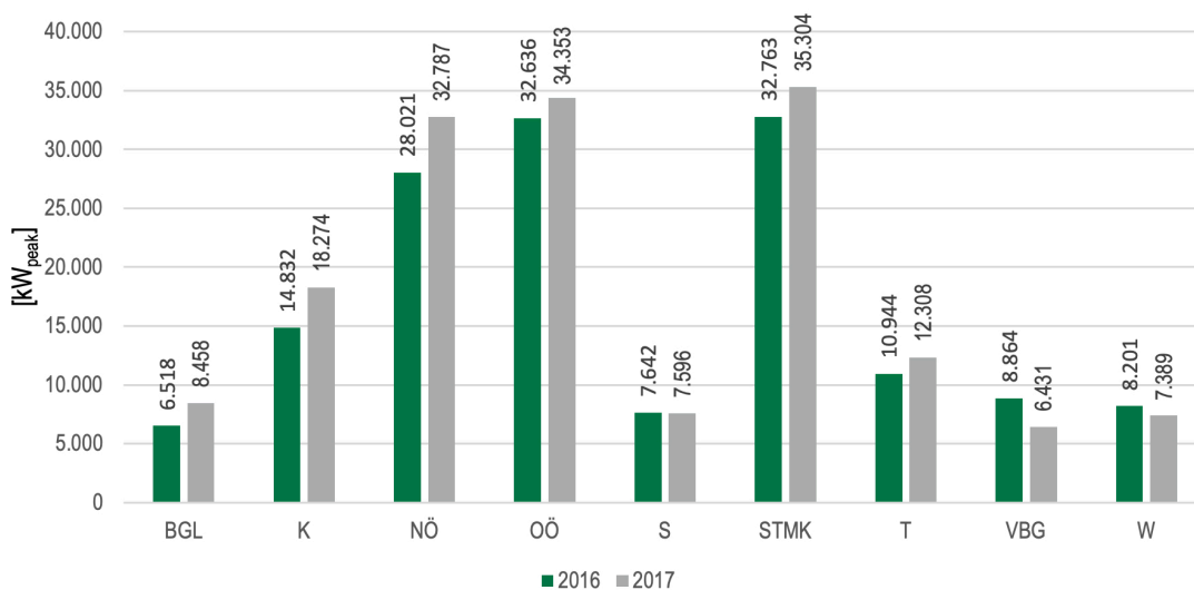
Abbildung 37: Geförderte PV-Anlagen nach Leistung im Bundesländervergleich [12]
