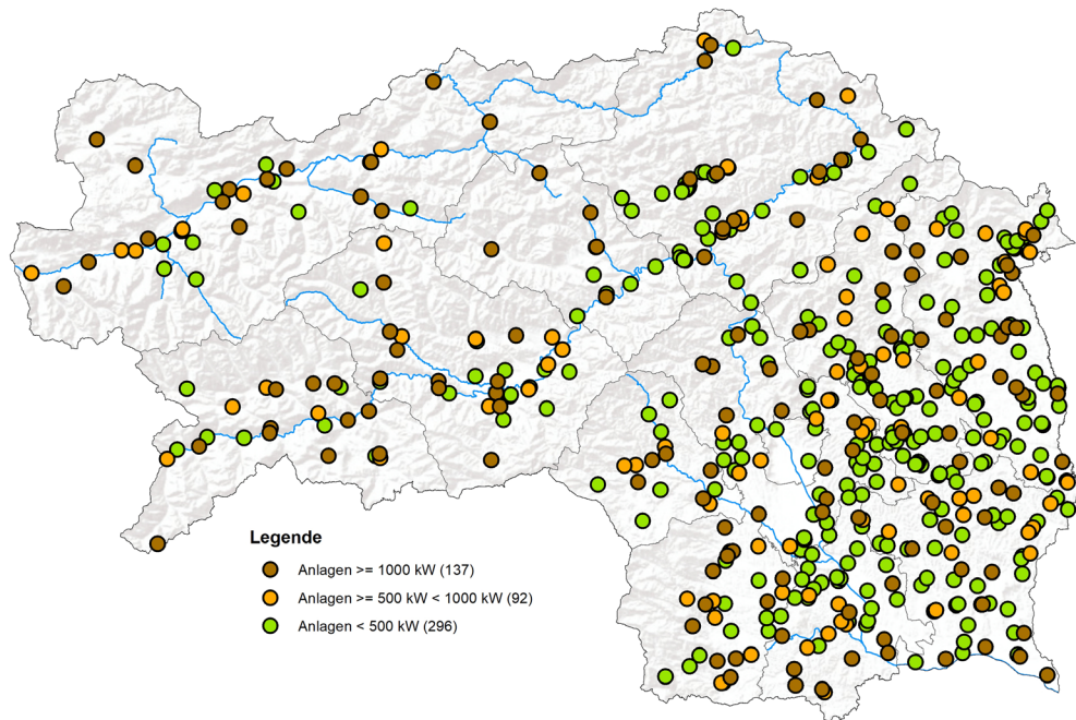
Abbildung 27: Biomasse-Heizwerke und KWK-Anlagen in der Steiermark (Stand 2017) [5]
