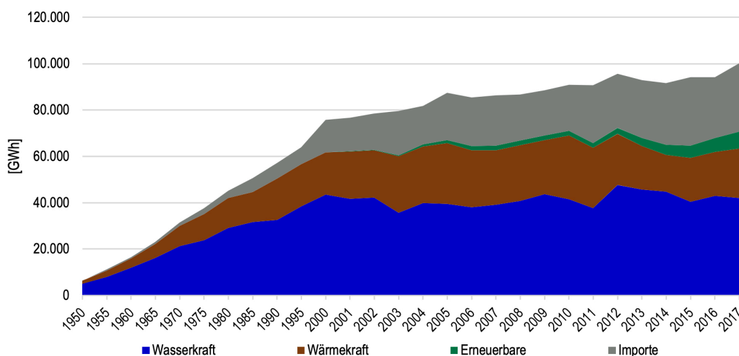
Abbildung 42: Entwicklung der Aufbringung elektrischer Energie in Österreich 1950–2017 in [GWh] [26] [16]
