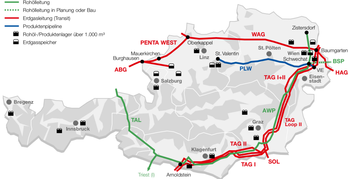
Abbildung 12: Erdöl- und Erdgasleitungen in Österreich und der Steiermark [22]
