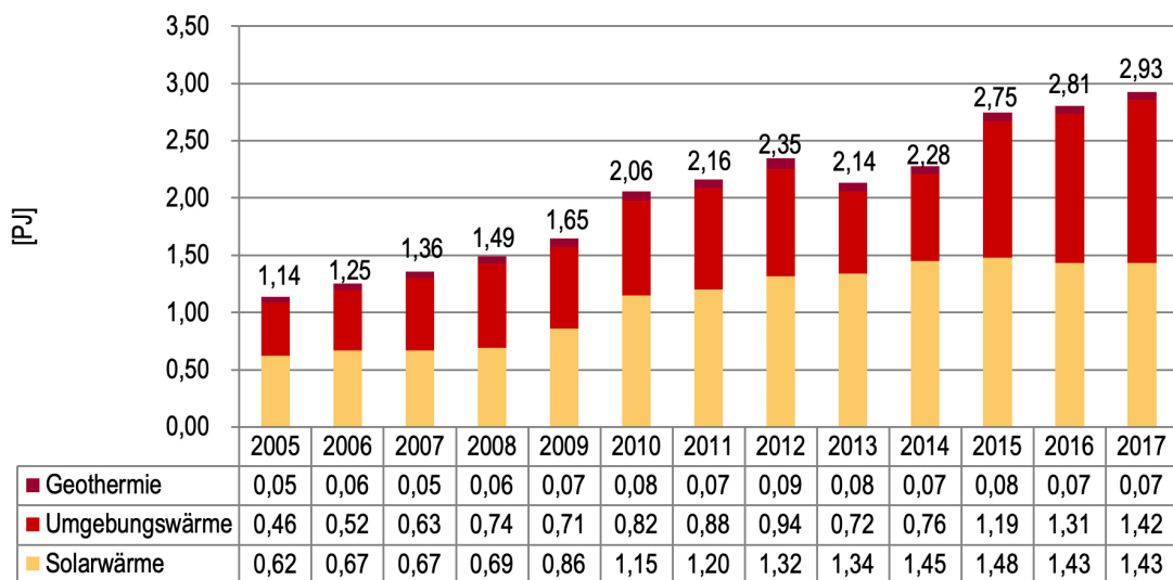
Abbildung 38: Energetischer Endverbrauch von Umgebungswärme in den Jahren 2005–2017 [30]
