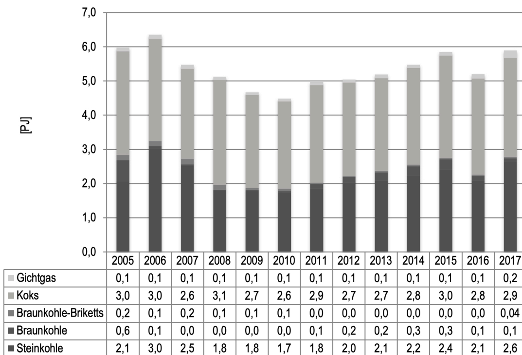
Abbildung 20: Energetischer Endverbrauch von Kohlen in den Jahren 2005–2017 in PJ [30]
