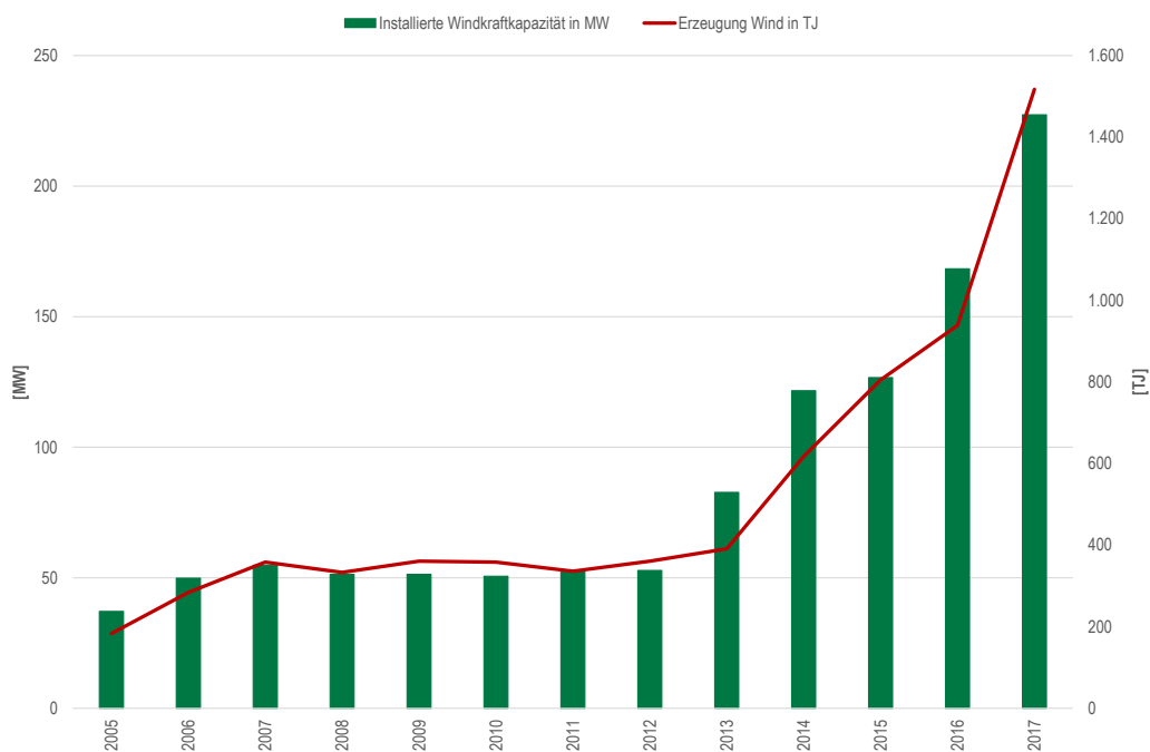
Abbildung 32: Entwicklung der installierten Leistung von Windkraftanlagen mit produzierter Energiemenge [30]
