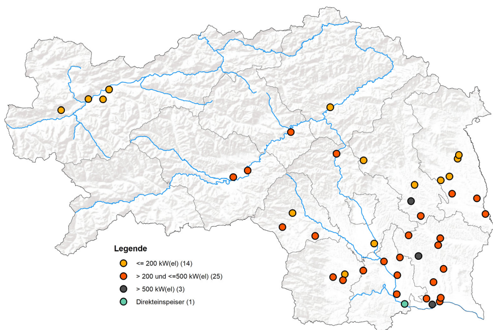
Abbildung 28: Biogasanlagen in der Steiermark (Stand 2014) [5]
