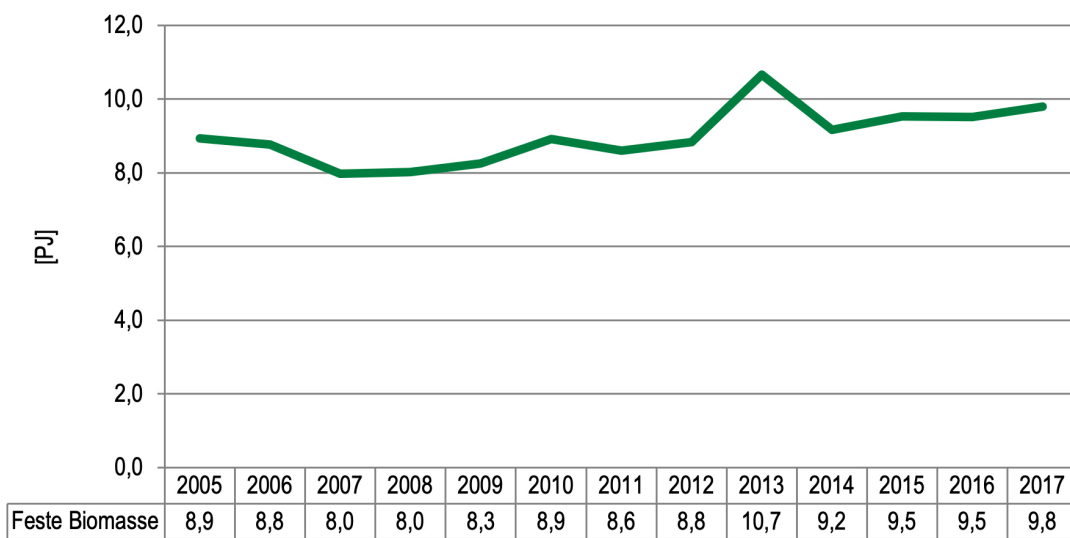
Abbildung 26: Energetischer Endverbrauch von fester Biomasse in den Jahren 2005–2017 in PJ [30]
