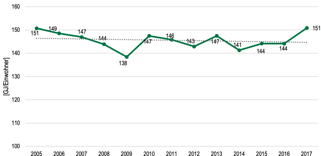
Abbildung 47: Entwicklung des energetischen Endverbrauchs je Einwohner in der Steiermark
