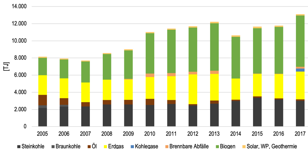
Abbildung 45: Energetischer Endverbrauch von Fernwärme in den Jahren 2005–2017 in TJ [30]
