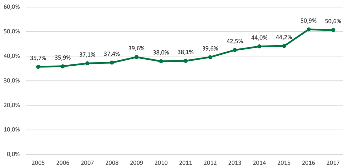
Abbildung 24: Entwicklung des Anteiles anrechenbarer erneuerbarer Elektrizitätserzeugung in der Steiermark nach EU-Definition [30]
