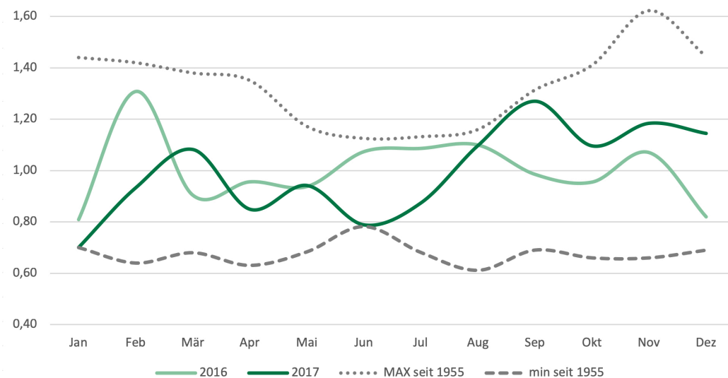
Abbildung 30: Entwicklung der Erzeugungskoeffizienten der Wasserkraft [18]
