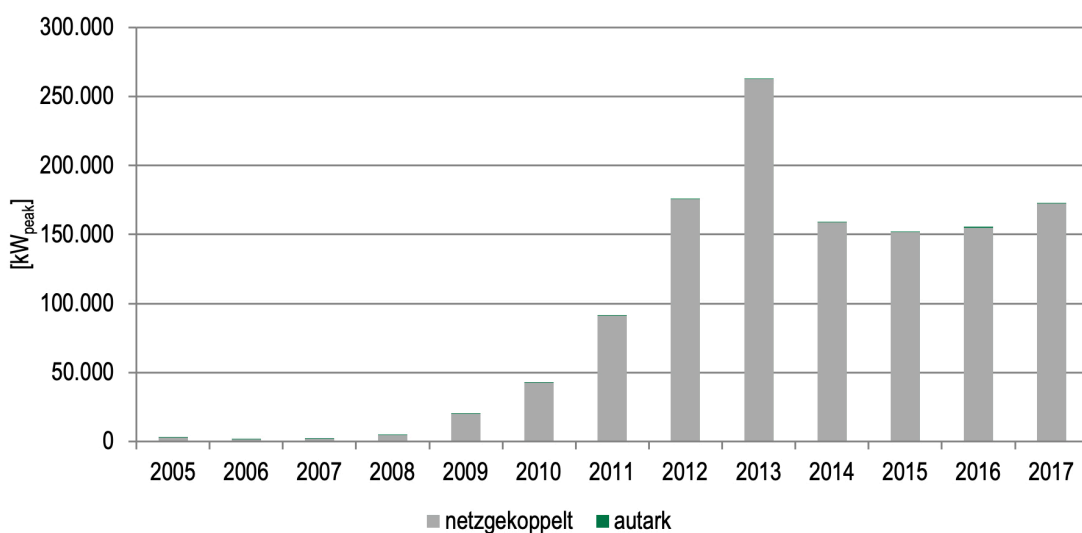
Abbildung 35: Entwicklung der jährlich installierten PV-Leistung in Österreich [12]
