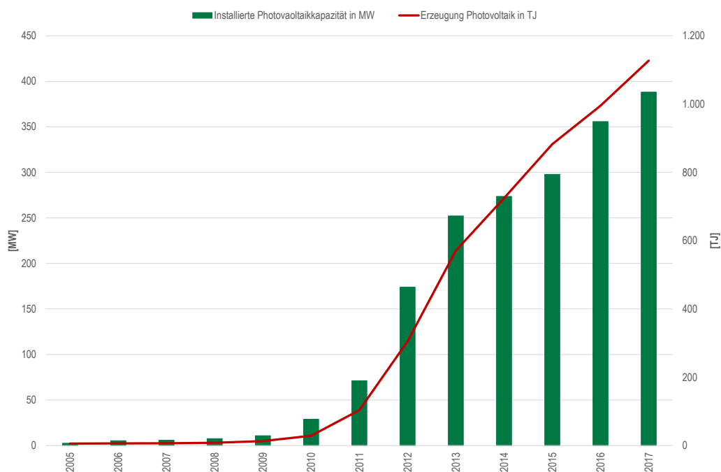
Abbildung 36: Entwicklung der anerkannten Leistung von PV-Anlagen mit produzierter Energiemenge [17, 30]
