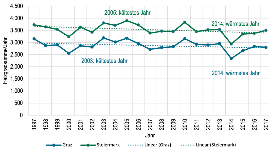
Abbildung 9: Entwicklung der Heizgradsummen für Graz und die Steiermark (Datenquelle: ZAMG Steiermark)
