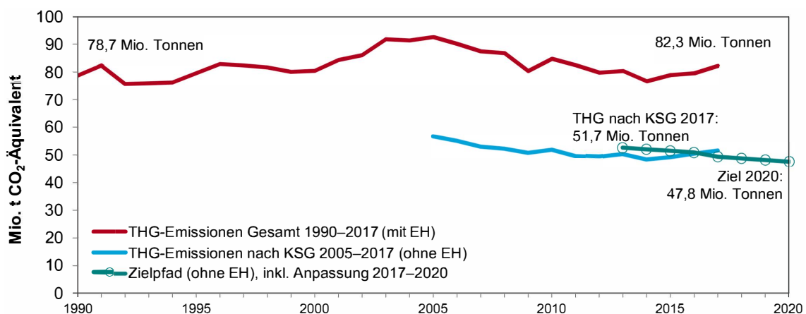
Abbildung 5: Verlauf der österreichischen THG-Emissionen 1990–2017 mit und ohne Emissionshandel (EH) und Zielpfad nach dem österreichischen Klimaschutzgesetz (KSG) [13]
