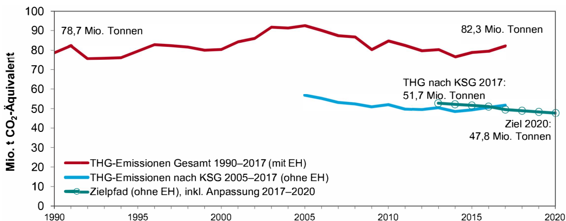
Abbildung 1: Verlauf der österreichischen THG-Emissionen 1990–2017 mit und ohne Emissionshandel (EH) und Zielpfad nach dem österreichischen Klimaschutzgesetz (KSG) [13]
