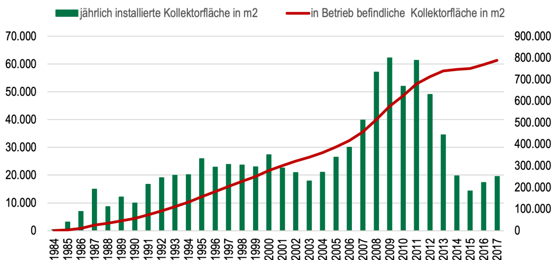
Abbildung 39: Entwicklung der installierten thermischen Kollektorfläche in der Steiermark [12]
