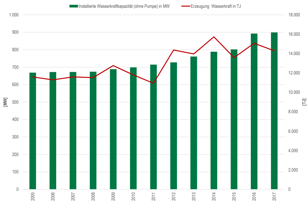
Abbildung 29: Entwicklung der installierten Leistung von Wasserkraftanlagen mit produzierter Energiemenge [30]
