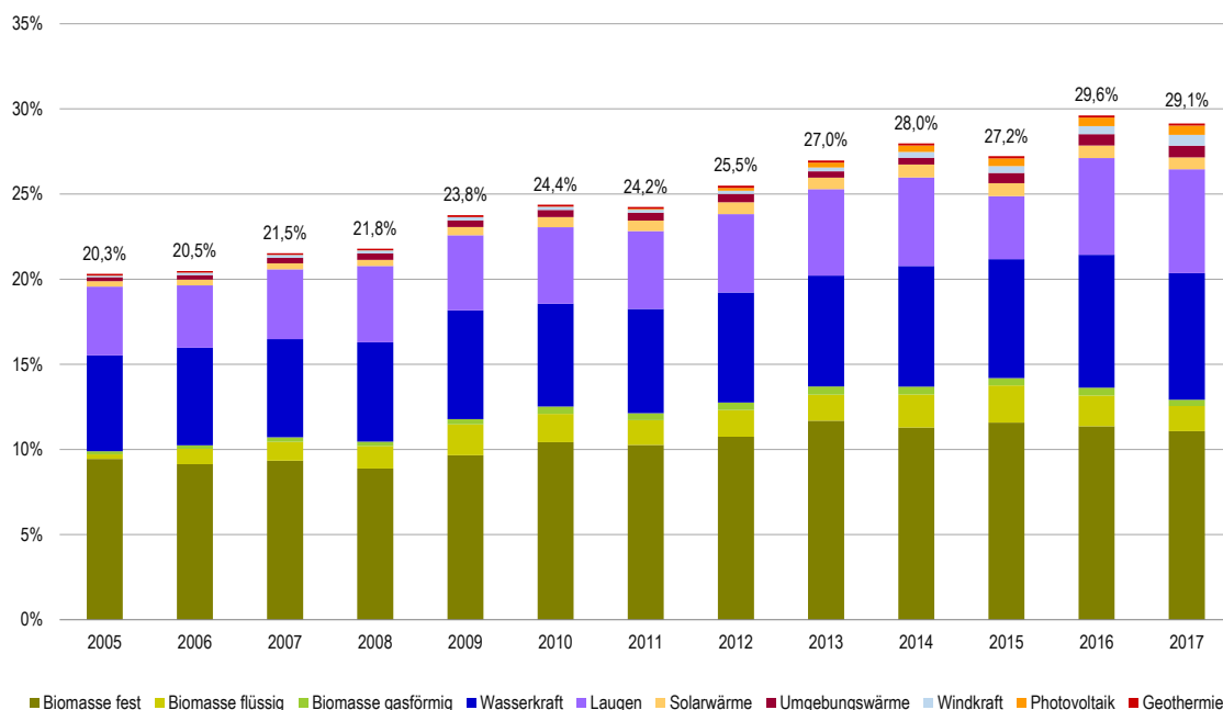
Abbildung 3: Entwicklung des Anteils anrechenbarer erneuerbarer Energien in der Steiermark 2005–2017 [30]
