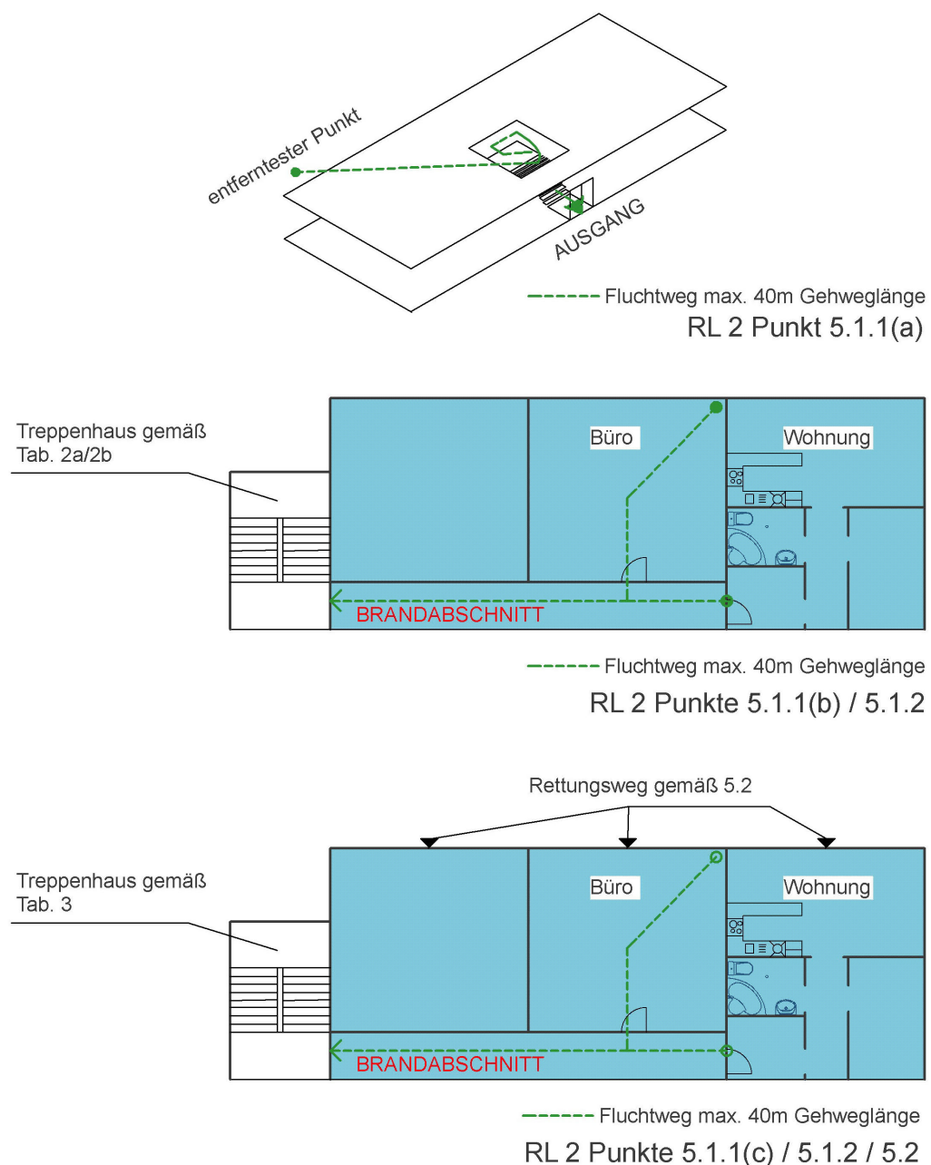
Abbildung 16: zu den Punkten 5.1 und 5.2 – Flucht- und Rettungswege – Übersicht
