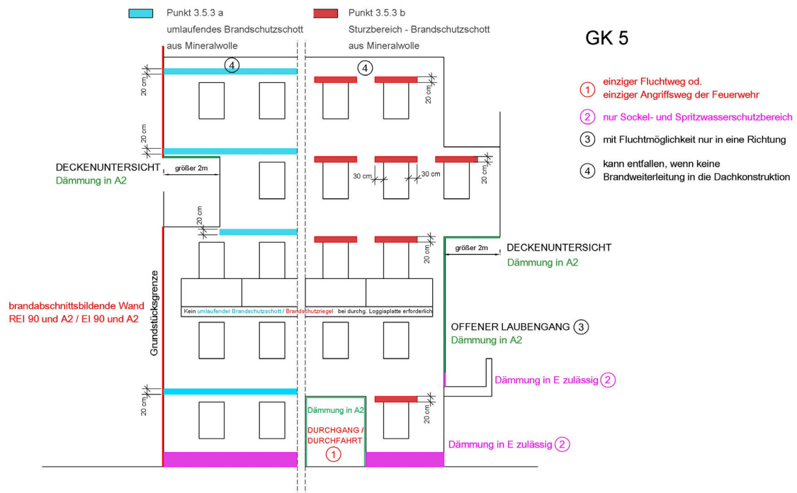
Abbildung 14: zu den Punkten 3.5.3, 3.5.4 und 3.5.5 – Zusammenstellung der Anforderungen an Außenwand-Wärmedämmverbundsysteme bei Gebäuden der GK 5
