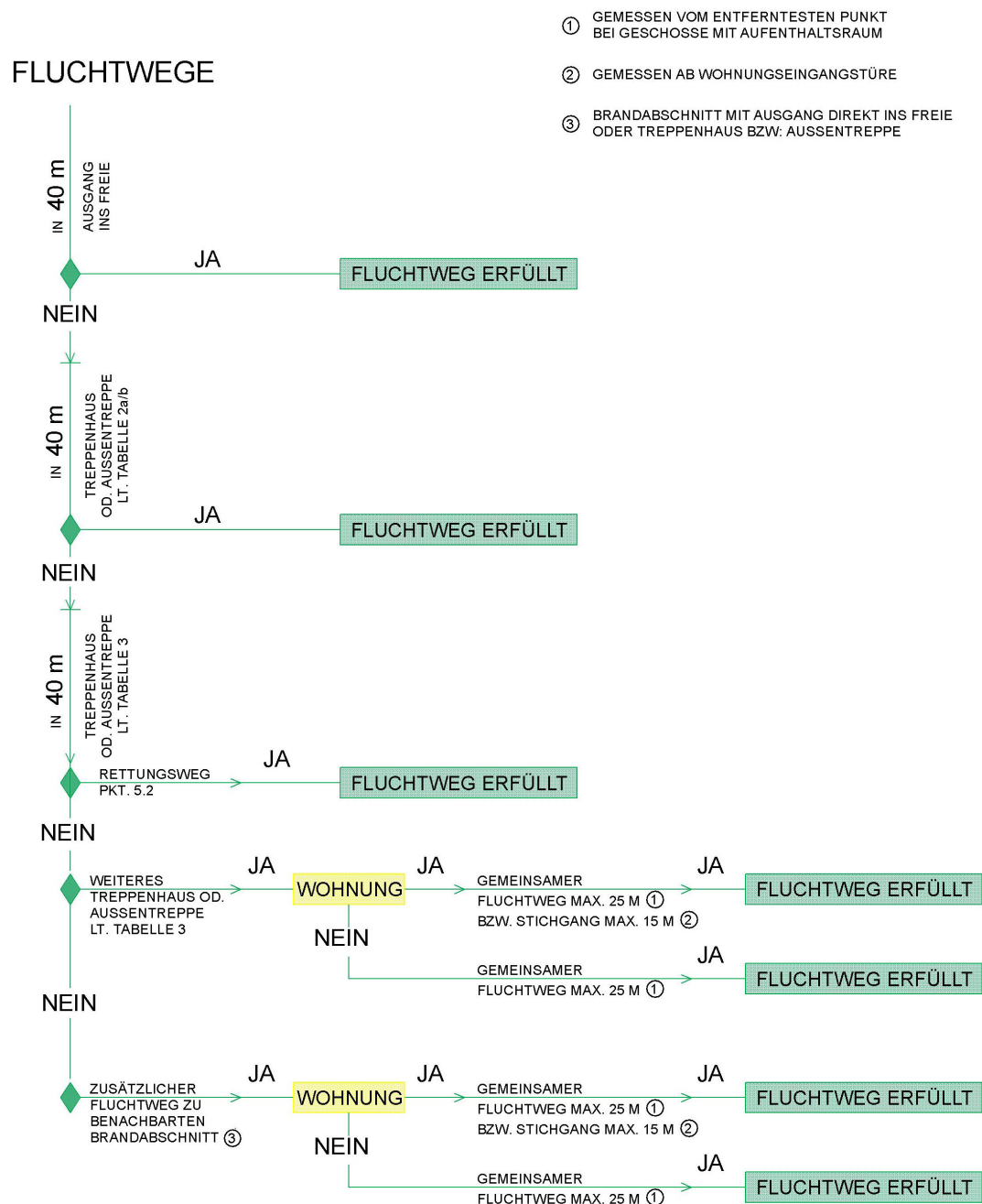
Abbildung 15: zu den Punkten 5.1 und 5.2 – Flucht- und Rettungswege – Ablaufschema
