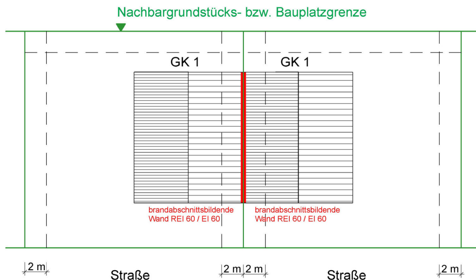
Abbildung 6: zu Punkt 3.1 der Tabelle 1b – zwei Gebäude der GK 1 an der Nachbargrundstücks- bzw. Bauplatzgrenze zusammengebaut
