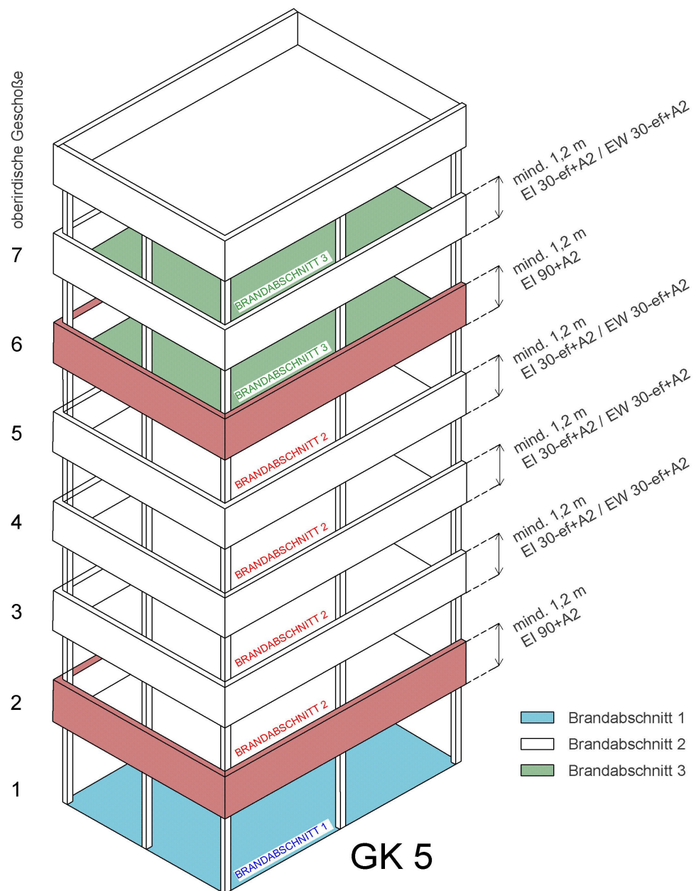
Abbildung 11: zu den Punkten 3.3 und 3.1.7 – deckenübergreifender Außenwandstreifen bei GK 5 bzw. Außenwandstreifen bei Brandabschnitten
